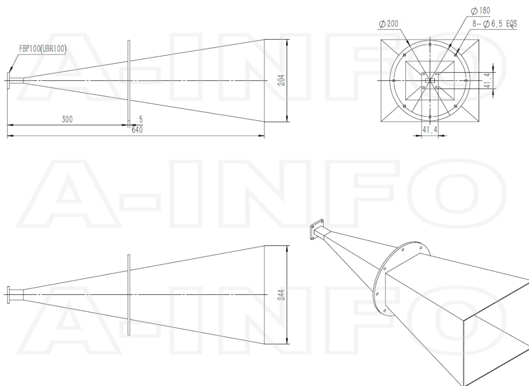
FBP100 Output (P/N: LB-90-25-A2)
